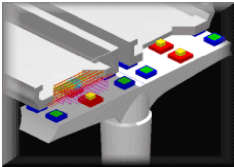
橋墩帽樑與預鑄樑
