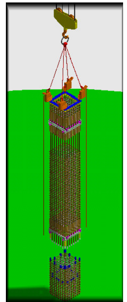
鋼筋籠吊裝流程動畫
