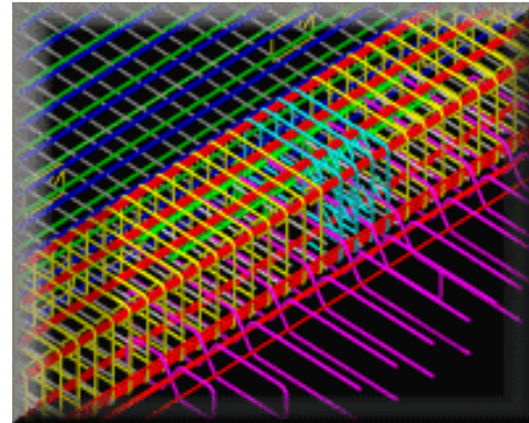
鋼筋組立細部
