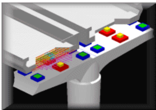
橋墩帽樑與預鑄樑
