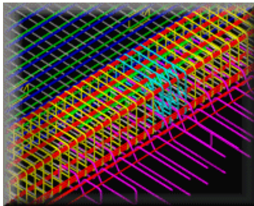
鋼筋組立細部
