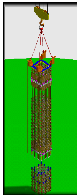
鋼筋籠吊裝流程動畫
